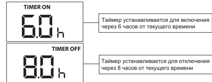
Дисплей пульта ДУ
