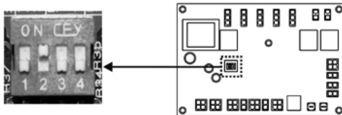
Управление электрическим предварительным нагревателем
