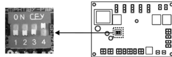
Функция внешнего мониторинга (BSM)
